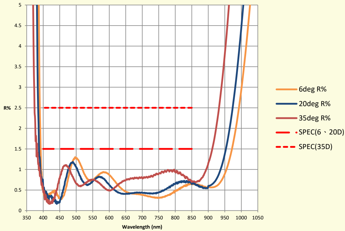
反射光譜 %
